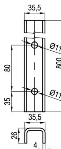
0354 200.200 Výztuha U 35,5x27-800mm Spojovací materiál je součástí dodávky
